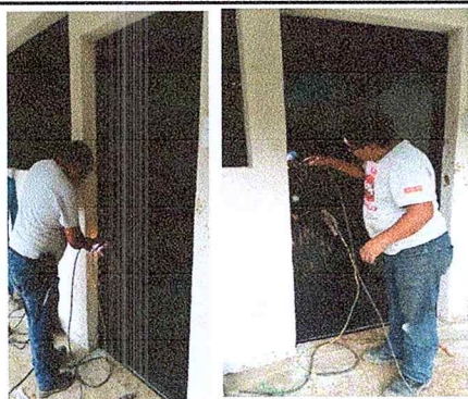
Foto 3: Mejoramiento de puertas de lámina por puertas prensadas de metal con su respectiva chapa.
